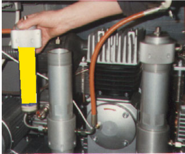
Abbildung : Entfernen des Ringdeckels und der Molekularsieb-Patrone
