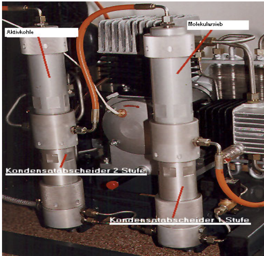
Abbildung : Filtersystem
