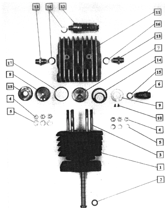
Abbildung : Ansicht Hochdruckkolben Hochdruckzylinder und Zylinderkopf der 3° Stufe
